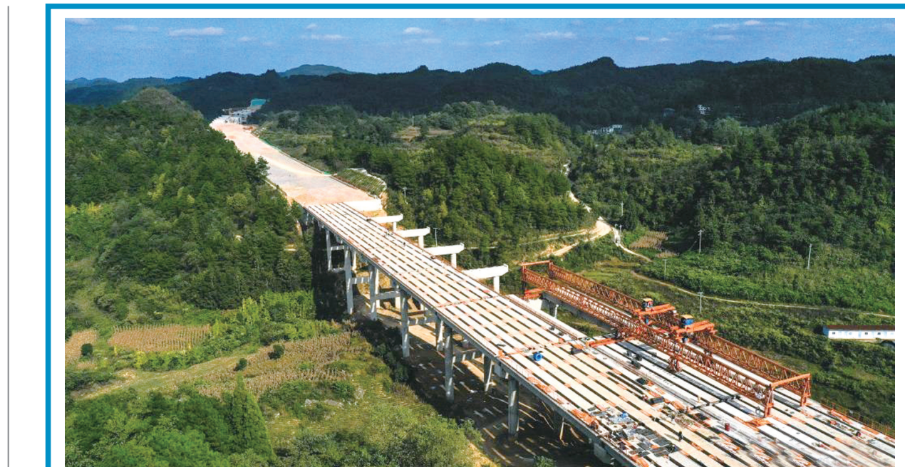
10月9日,中铁二十局的工人在贵州乌当高速1标段穿洞大桥上施工(无人机照片)。目前,贵州乌当至长顺高速公路建设现场的工人们正加紧架设桥梁、修筑边坡、铺设路面,全线建设正有序推进。乌当高速公路起于贵阳市乌当区,止于长顺县,全长约115公里,设计为双向六车道,时速100公里。建成后将成为连通兰海、沪昆、银百等国家高速公路的便捷大通道,对于促进黔南地区经济社会发展具有重要意义。
